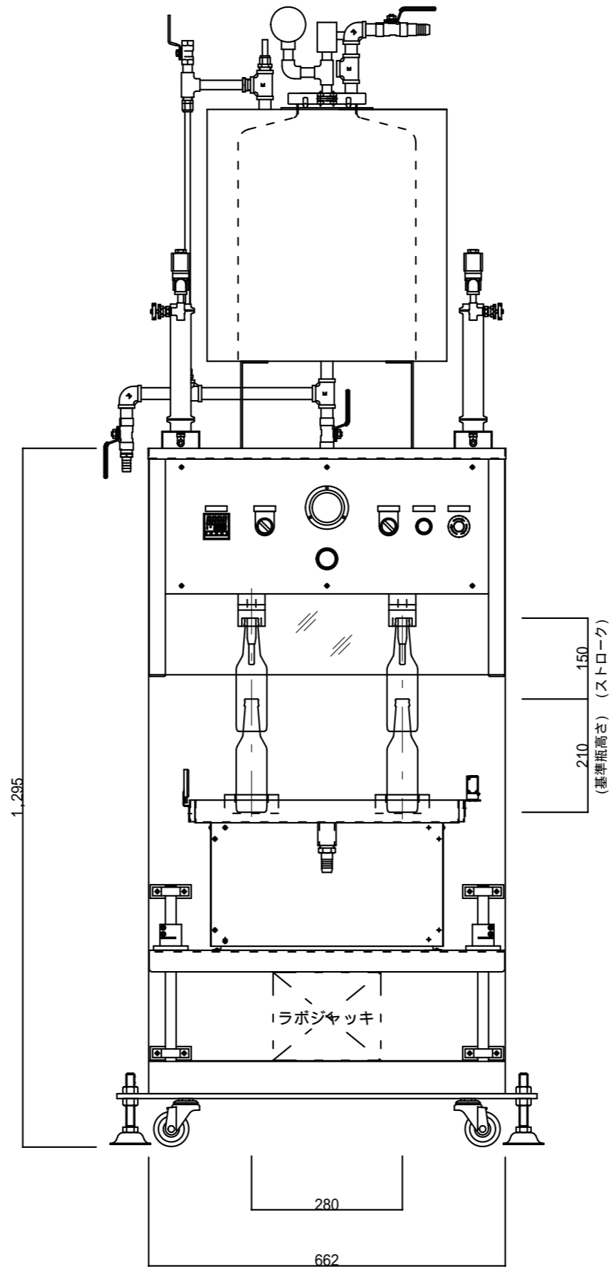
立面図 1/10
